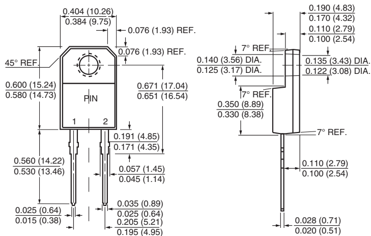
ITO-220AC
