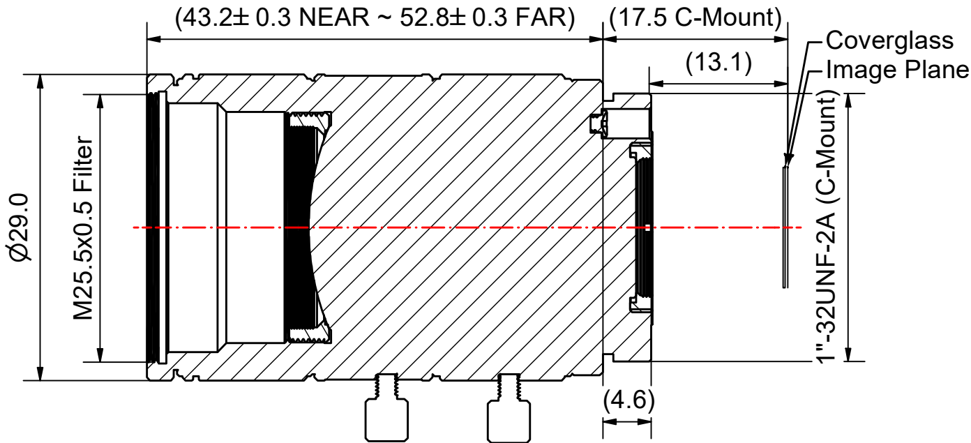
A-A ( 2 : 1 )
