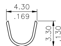
SEC: A-A
