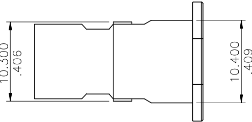
Wedgelock
