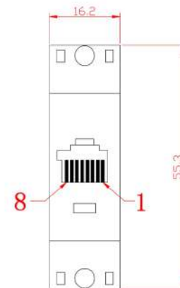
RJ45
