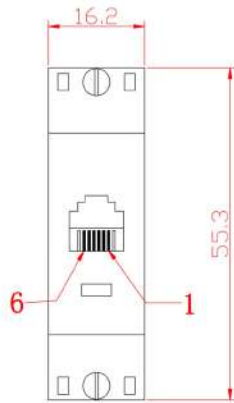
RJ12
