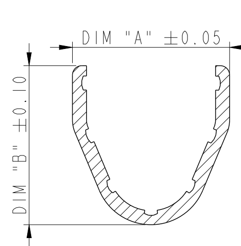
SECTION AA-AA SCALE 25:1
