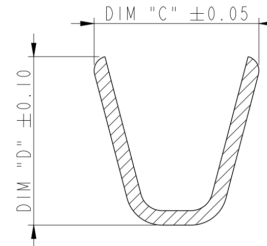
SECTION AB-AB SCALE 25:1
