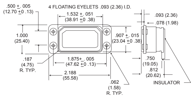
DPAF-34
