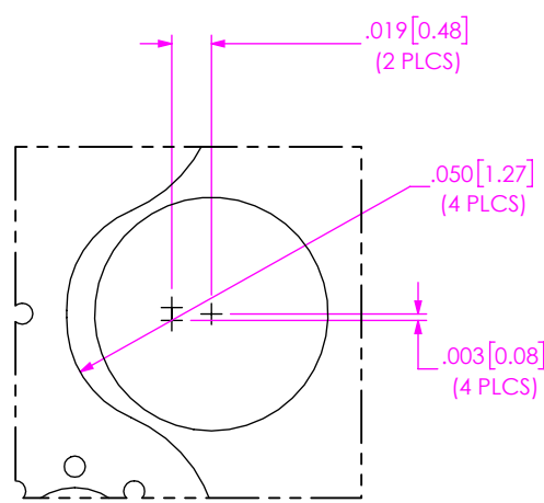
DETAIL 'B' SCALE 10:1
