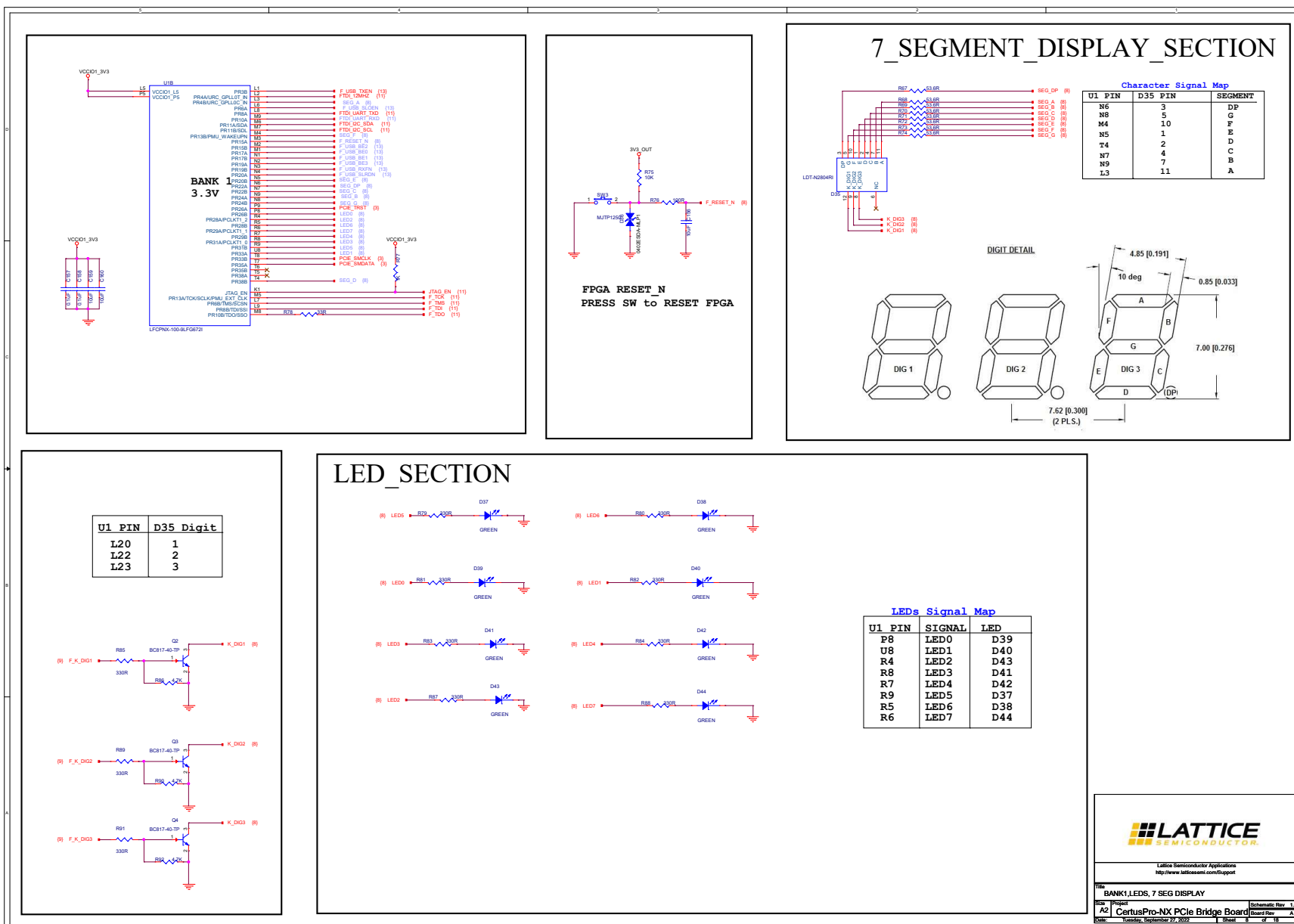
Figure A. 8. BANK1,LEDS, 7 SEG DISPLAY
