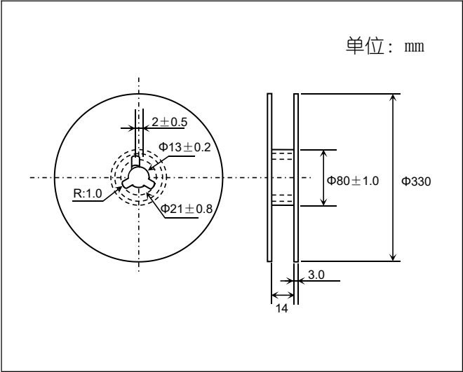
卷盘 Reel
