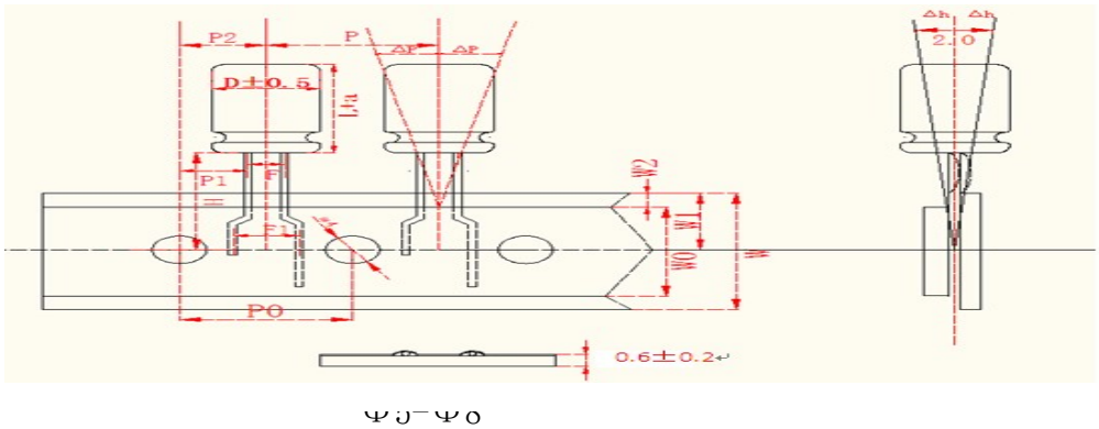
编带外型尺寸 B 图
