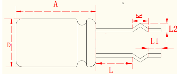
引线切脚成型 C 图
