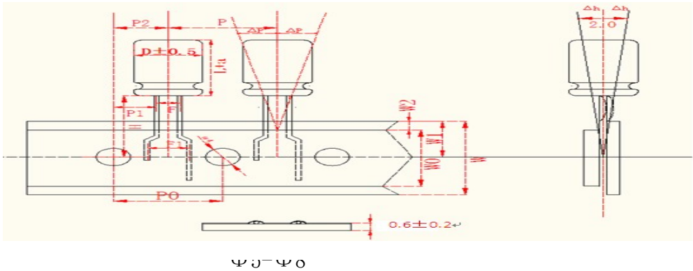
编带外型尺寸 B 图
