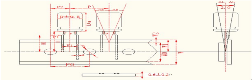
编带外型尺寸 A 图
