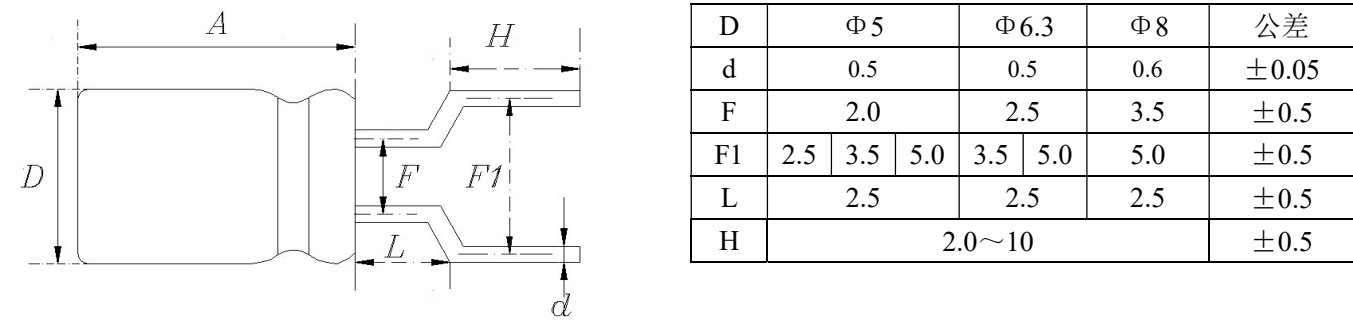
引线切脚成型 G 图
