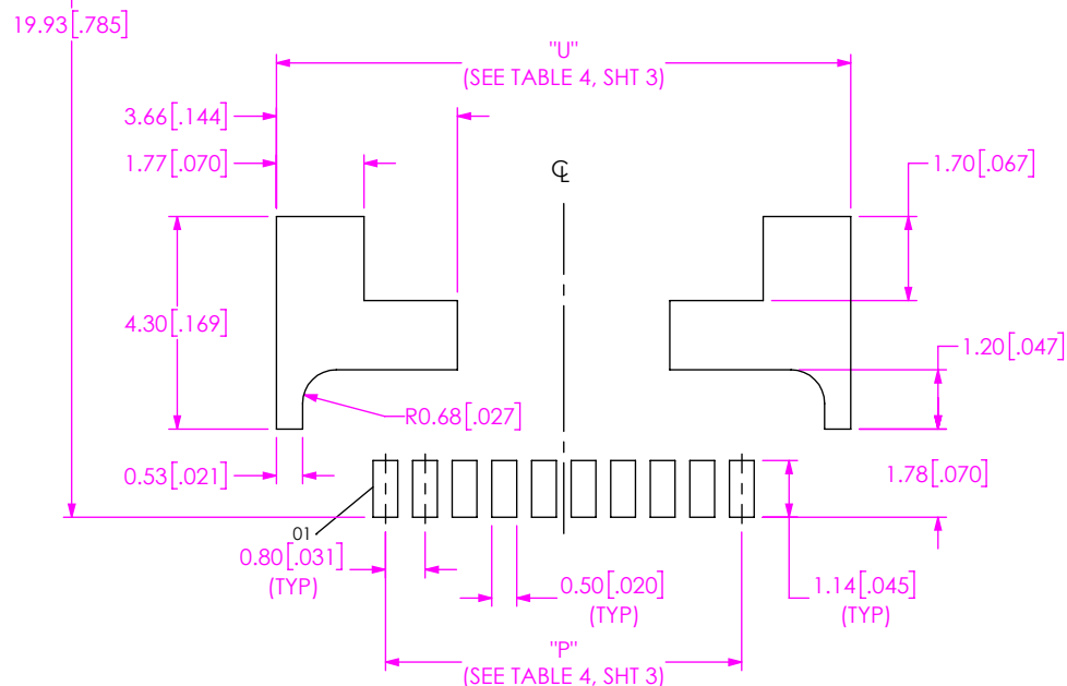
FIG 5 UEC5-019-1-X-D-RA-1-X STENCIL SHOWN UCC8-010-X-X-S-1-A STENCIL SHOWN
