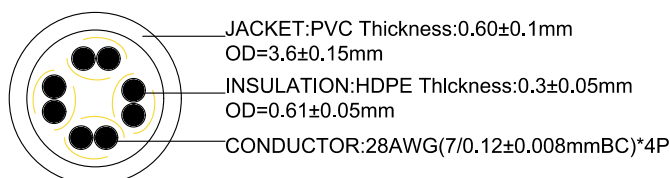
SEC:A-A
