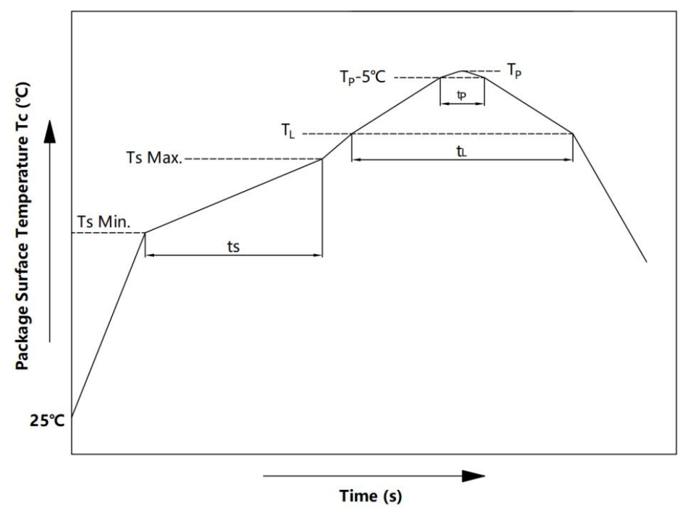
回流焊温度曲线图 Solder Reflow Profile
