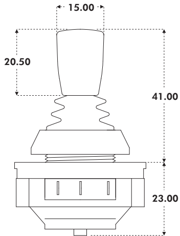
V4 DI-POLE
