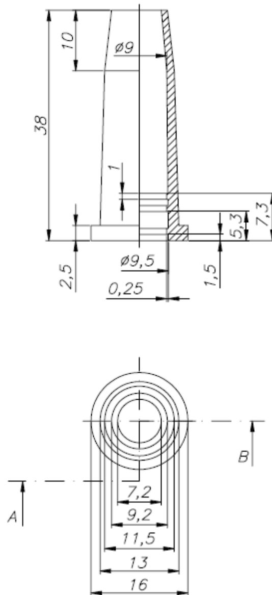
Schnitt A-B
