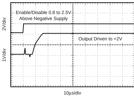
ENABLE ( 1\Omega Load)
