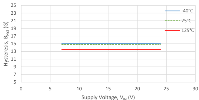
Hysteresis ( B_{HYS} v. V_{IN} )
