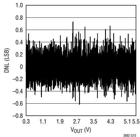
VOUT_COMMAND DNL
