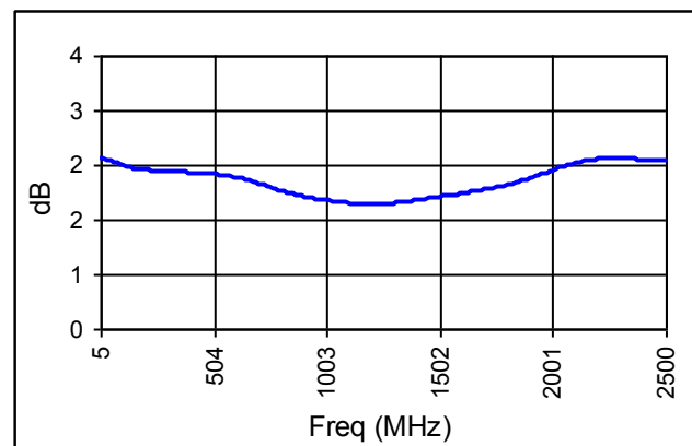
LO VSWR
