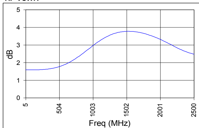
RF VSWR
