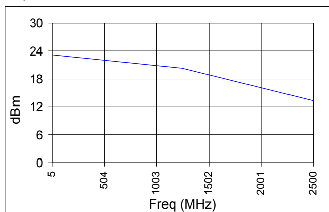
IP3
